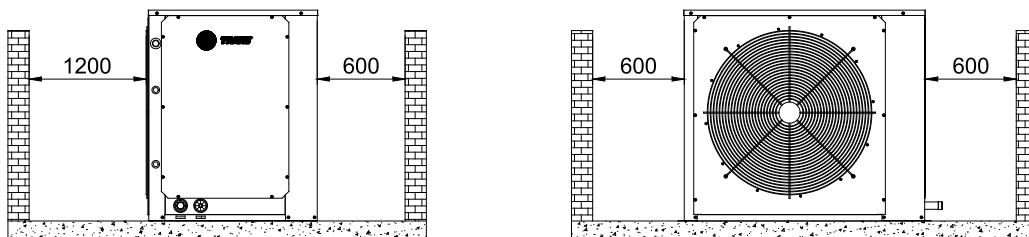
Fig. XVIII 40 - Espacios sugeridos TRAE 200 a 300 - Descarga Vertical
