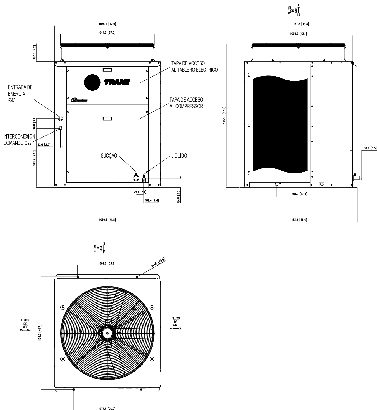
Fig. XI-31 - Dimensional Unidades Condensadoras TRAE 200 - 1 Circuito
