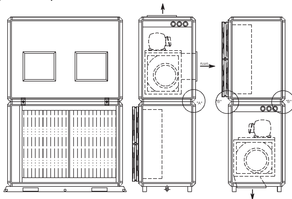
Fig. XI-15 - Montaje vertical 05 hasta 50 - DX/DL
