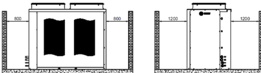
Fig. XI 41 - Espacios sugeridos para mantenimiento y circulación de aire. Unidad condensadora TRCE 050 a 150.
