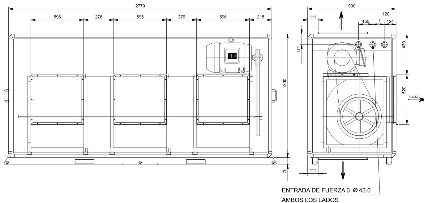
Fig. XI -08 - Dimensiones Módulo Ventilador 35/40/50 - Backward-Curved
