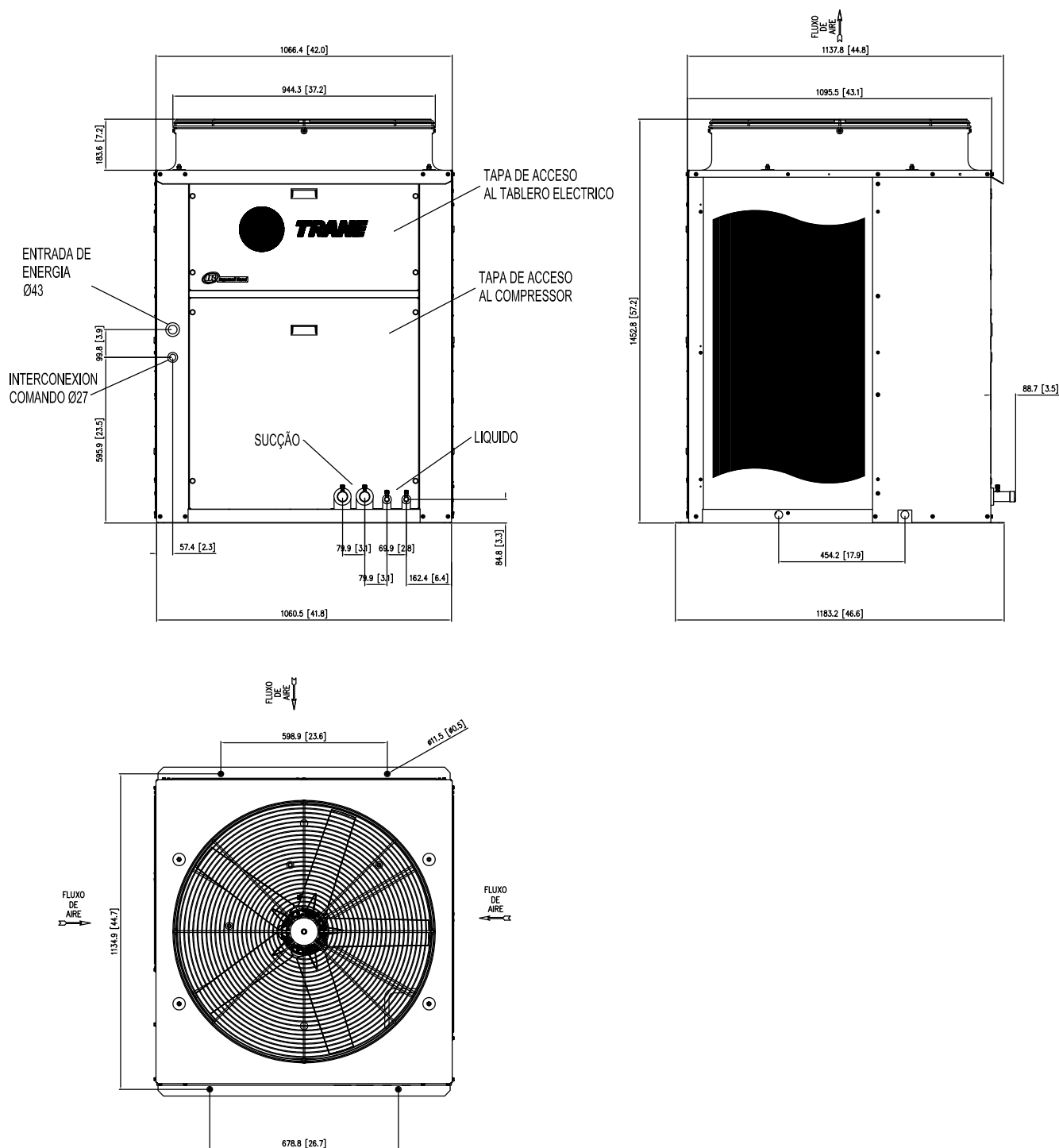
Fig. XI-32 - Dimensional Unidades Condensadoras TRAE 200 - 2 Circuitos
