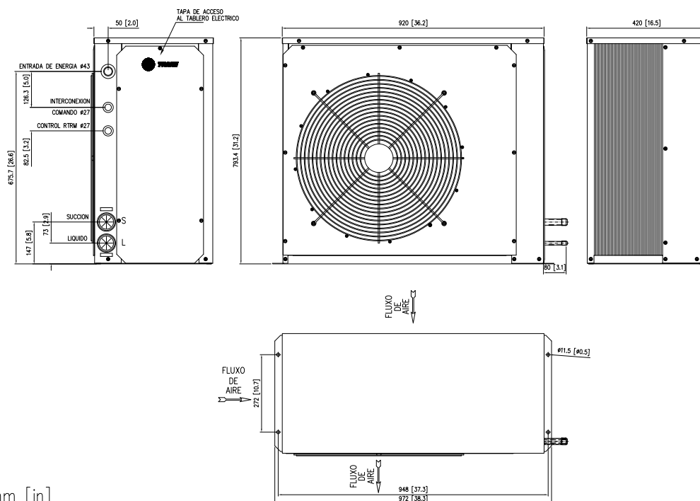
Fig. XI-25 - Dimensional Unidades Condensadoras TRAE 075 - 1 circuito
