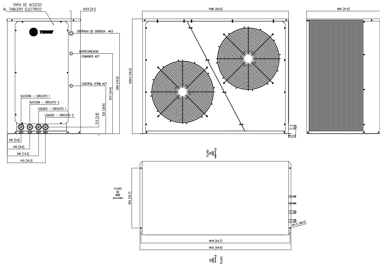
Fig. XI-30 - Dimensional Unidades Condensadoras TRAE 150 - 2 Circuitos
