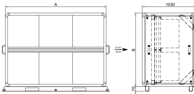
Fig. XI 03 - Cotas Módulo Filtro de Retorno - F8 Bolsa + 1" o solamente F8 Bolsa (12 hasta 50) Forward-Curved y Backward-Curved
