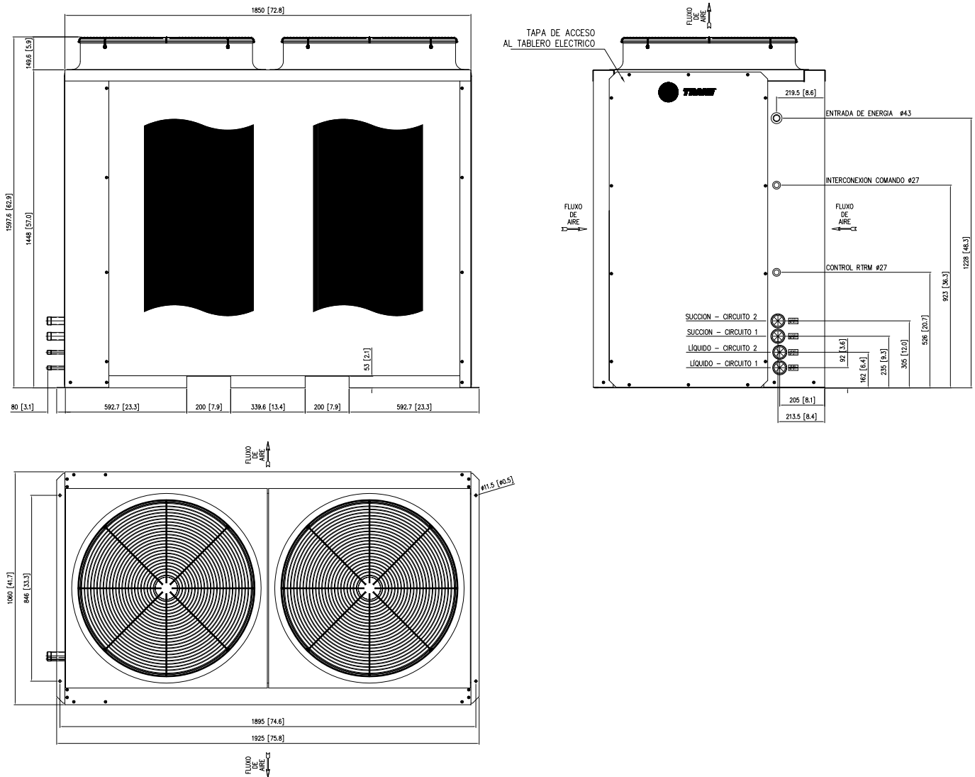
Fig. XI-35 - Dimensional Unidades Condensadoras TRAE 300 - 2 Circuitos
