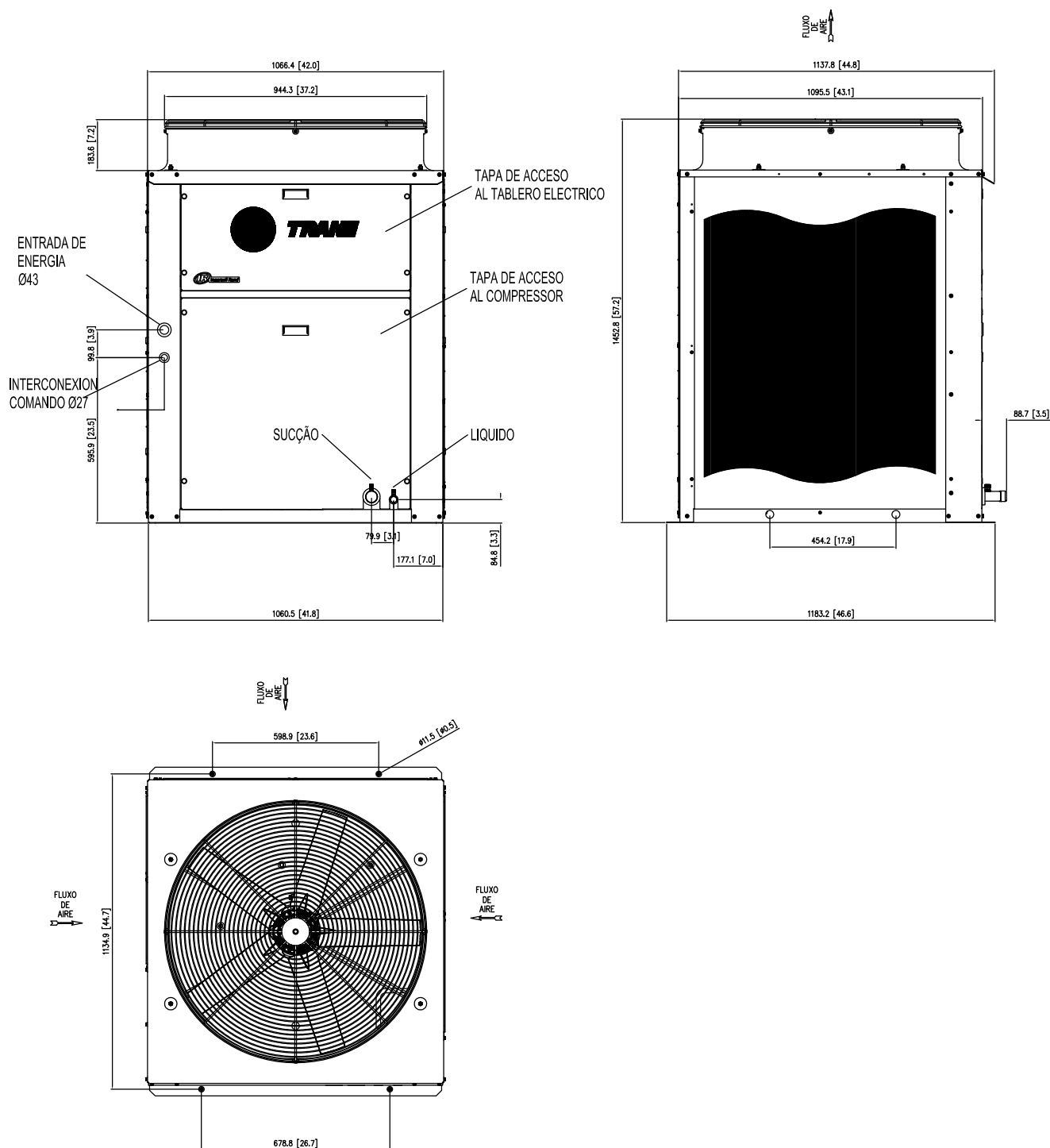
Fig. XI-33 - Dimensional Unidades Condensadoras TRAE 250 - 1 Circuito
