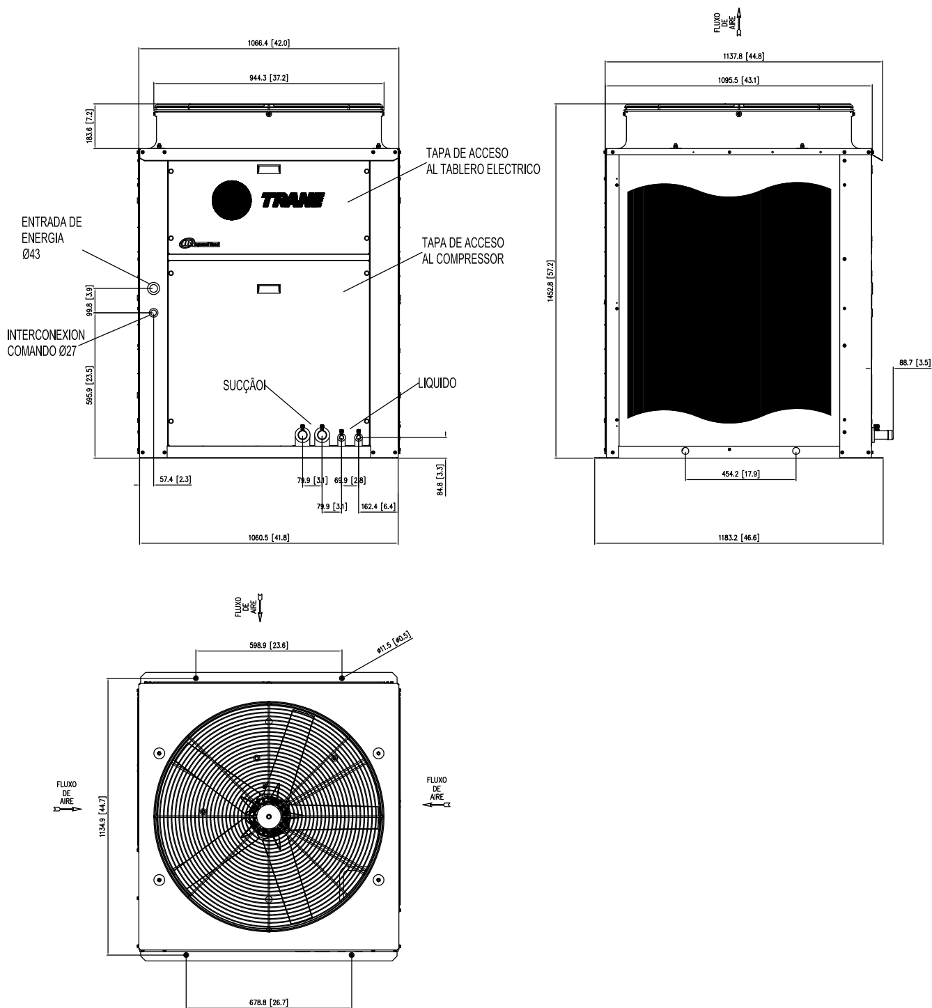
Fig. XI-34 - Dimensional Unidades Condensadoras TRAE 250 - 2 Circuitos
