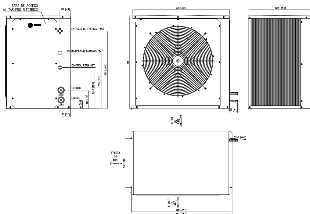
Fig. XI-25 - Dimensional Unidades Condensadoras TRAE 075 - 1 circuito
