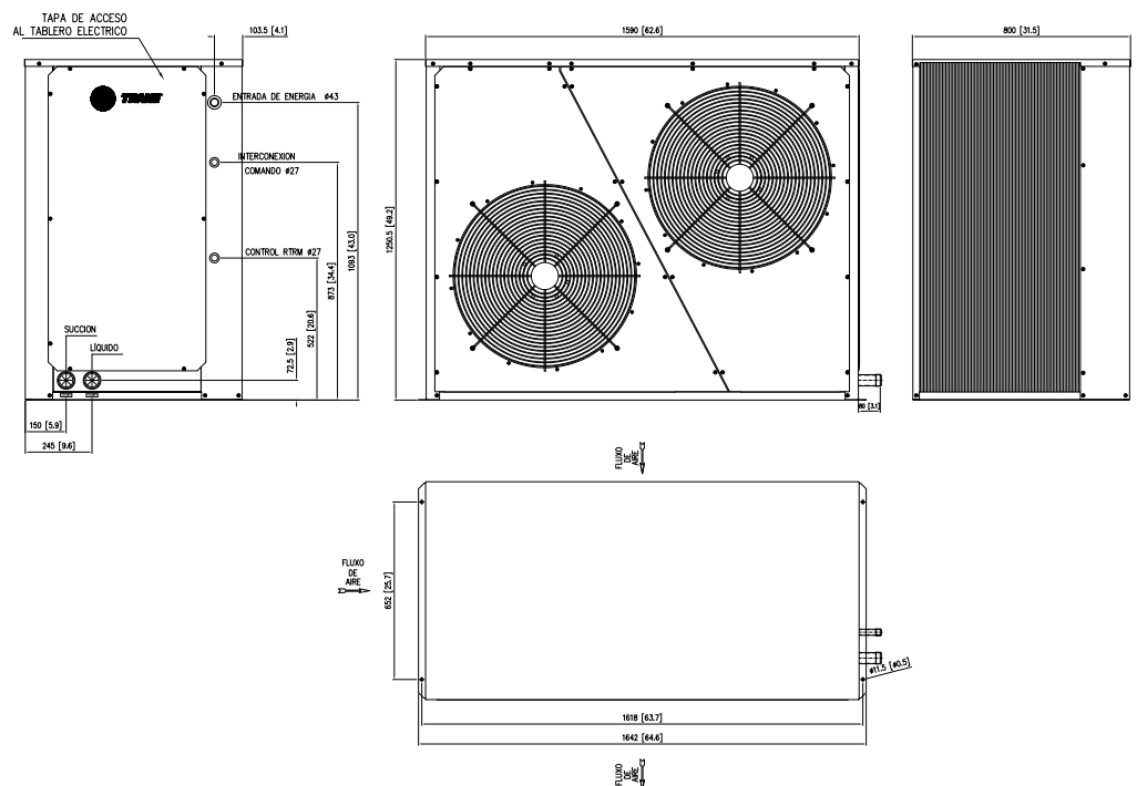
Fig. XI-29 - Dimensional Unidades Condensadoras TRAE 150 - 1 Circuito
