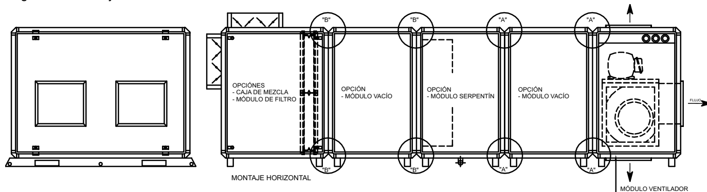
Fig. XI-16 - Montaje horizontal 05 hasta 50 - DX/DL
