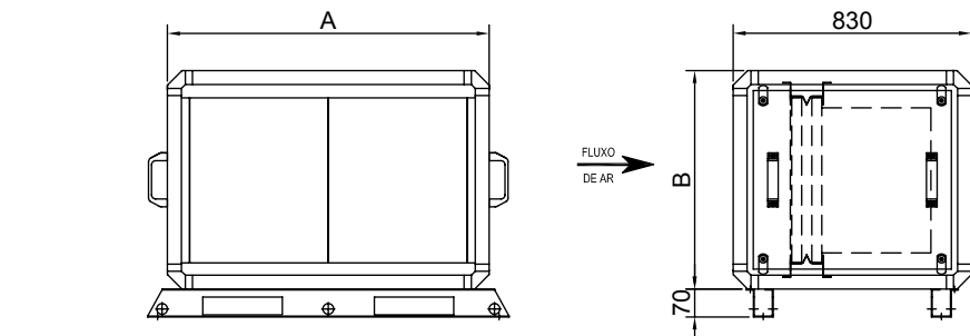
DADOS DIMENSIONAIS MÓDULO WD02 A WD 08 SIROCO
